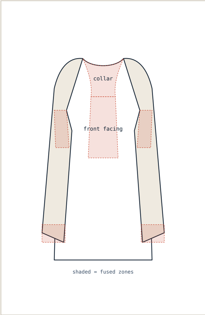
FUSING MAP · INT-004 WEFT INSERT
